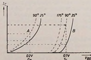
Fig. 3. I_c als functie van V_{BE} voor zowel een Ge (A) als voor een Si (B) transistor.
